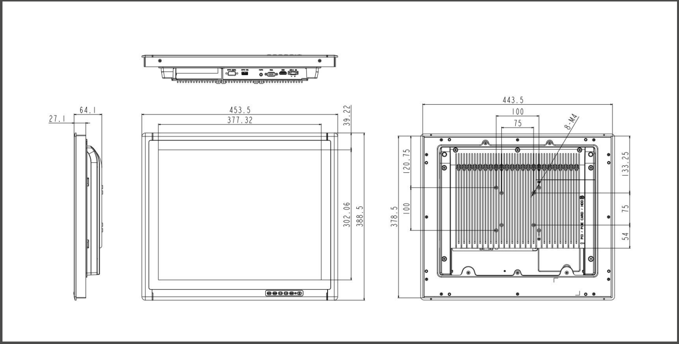
尺寸图 单位:mm
